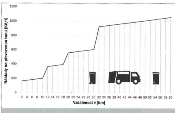
Obrázek 2: Závislost nákladů na dopravu SKO pro různé nájezdové vzdálenosti
