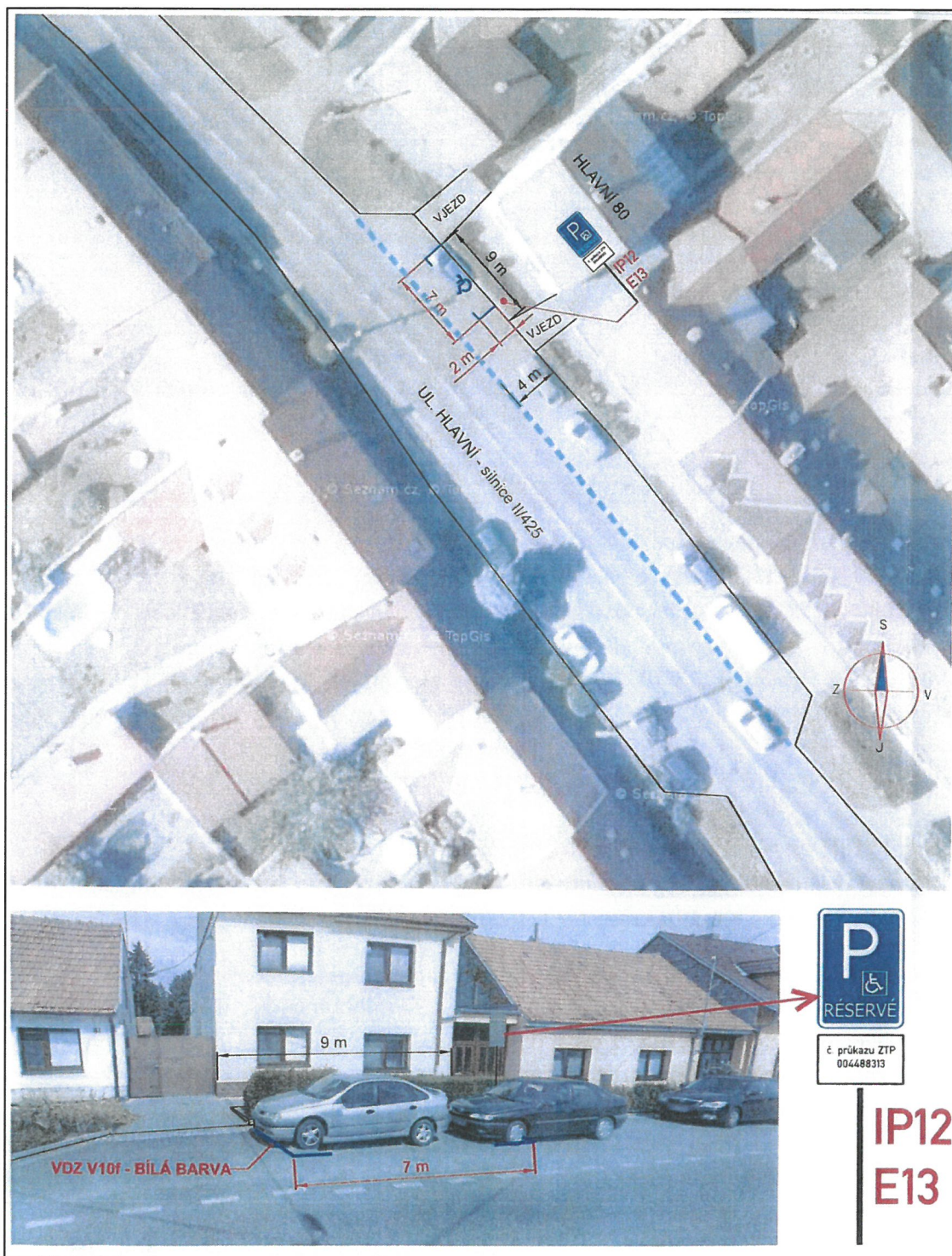
Obr. 1 – Výkres situace
